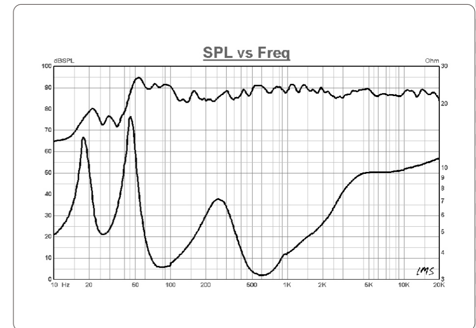
DX-7 频率响应 / 阻抗曲线图
